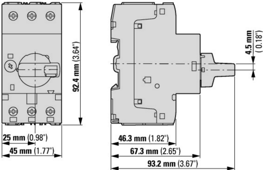
Wyłącznik silnikowy z zamykanym pokrętle PKZM0-...+AK-PKZ0
