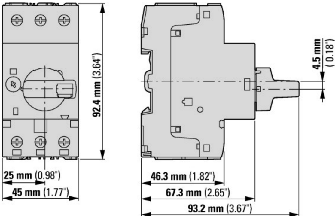
Wyłącznik silnikowy z zamykanym pokreplem PKZM0-...+AK-PKZ0
