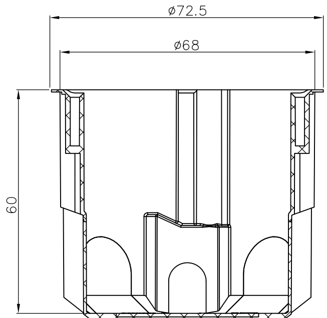
PRZEKRÓJ A-A SKALA 1 : 1
